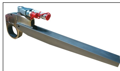
Abstützverlängerung
